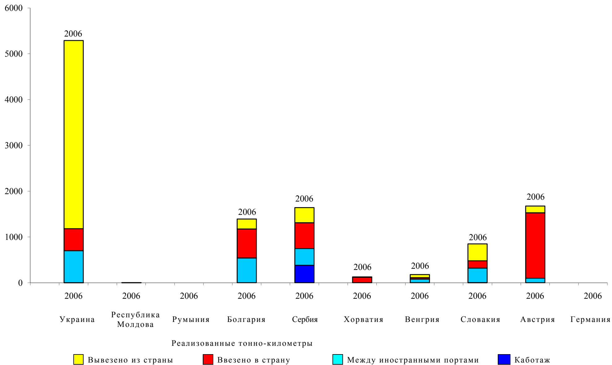
Рисунок IV.3 ТОННО-КИЛОМЕТРОВАЯ ПРОДУКЦИЯ, РЕАЛИЗОВАННАЯ НАЦИОНАЛЬНЫМИ СУДАМИ СТРАН-ЧЛЕНОВ ДУНАЙСКОЙ КОМИССИИ В 2006 г.
