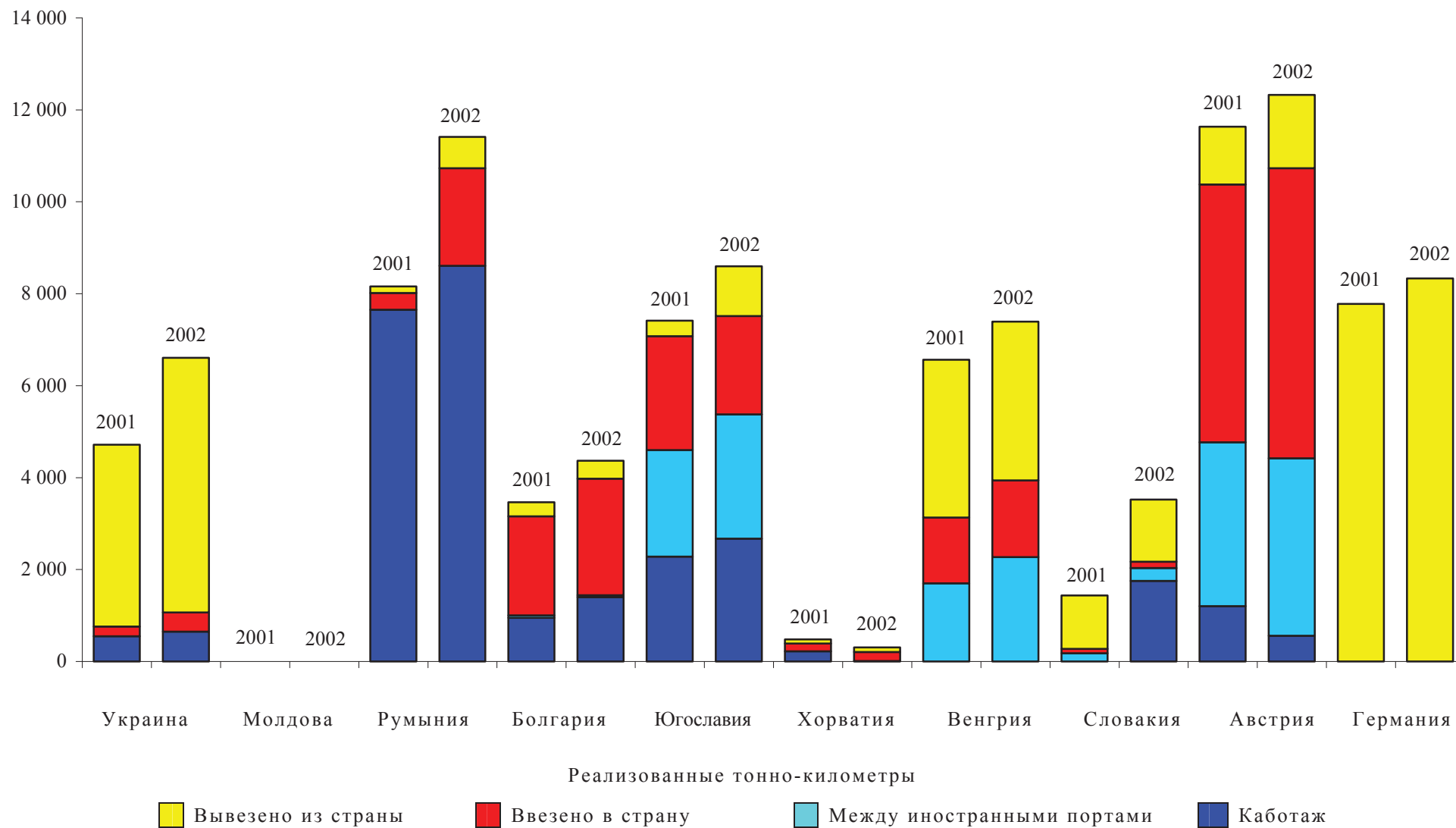
Рисунок III.3 ТОННО-КИЛОМЕТРОВАЯ ПРОДУКЦИЯ, РЕАЛИЗОВАННАЯ НАЦИОНАЛЬНЫМИ СУДАМИ ПРИДУНАЙСКИХ СТРАН В 2002г.
