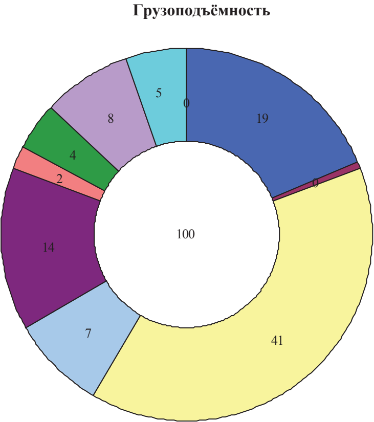
Рис. II.1 ОБЩАЯ ГРУЗОПОДЪЁМНОСТЬ И ОБЩАЯ МОЩНОСТЬ ДУНАЙСКОГО ФЛОТА ПО СТРАНАМ В 2002 году (%)
