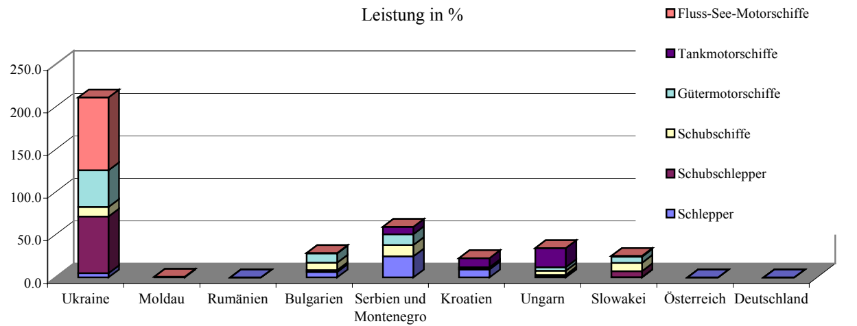
Abbildung II.4 FLOTTENBESTAND AUF DER DONAU NACH SCHIFFSGATTUNGEN, GRÖSSENKLASSEN TRAGFÄHIGKEIT UND MASCHINENLEISTUNG
